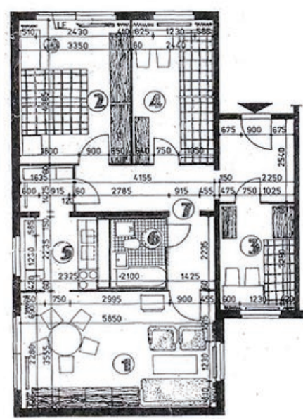
4-Raum-Wohnung 79,56 m 2
