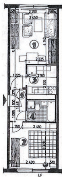
2-Raum-Wohnung 39,26 m 2
