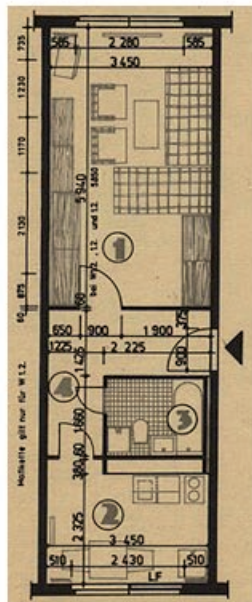
1-Raum-Wohnung 39,26 m 2
