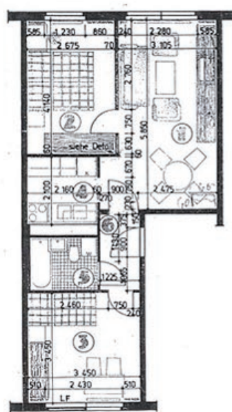
3-Raum-Wohnung 53,02 m 2
